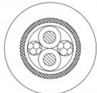
Sección transversal
