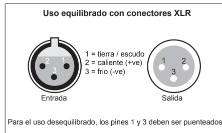
Fig. 3.1: Conexiones XLR
