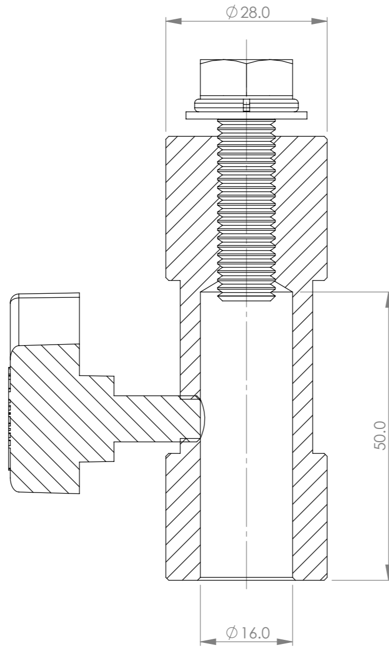
SECTION A-A
